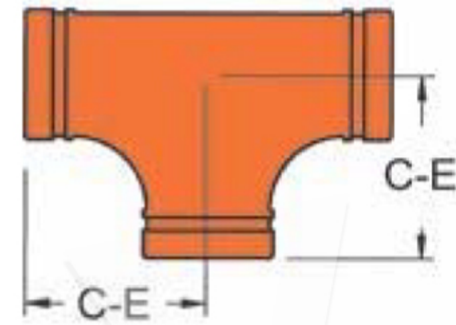
7120 Tee
